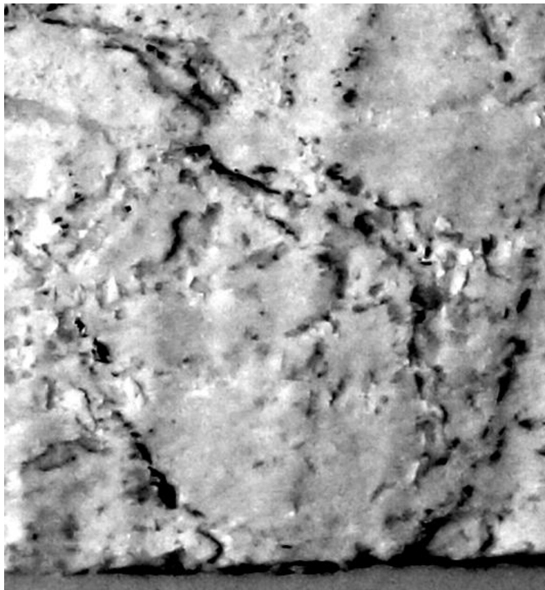
Рис. 3.46. Горизонтальный срез в нижней части образца 4 см от штуцера подачи газа. Образец с газом. Фото А.Н. Хименкова.
