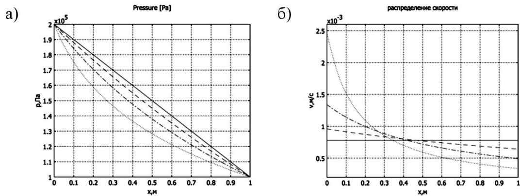
Рис. 6.23 Распределение давления и скорости на момент времени t = 1,0 c ; сплошная линия – \beta = 0 ; штриховая линия – \beta = 0,4 \cdot 10^{-5} Pa^{-1} ; штрих-пунктир – \beta = 1,0 \cdot 10^{-5} Pa^{-1} ; пунктир – \beta = 2,0 \cdot 10^{-5} Pa^{-1} .
