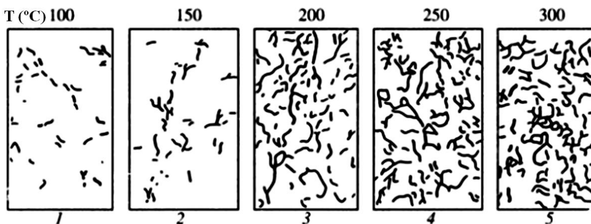
Рис. 3.5. Развитие межзерновой трещиноватости в образцах амфиболита при повышении температуры, постоянном гидростатическом давлении 180 МПа и постоянной сжатии 45 МПа [Абдрахимов и др., 1992].
