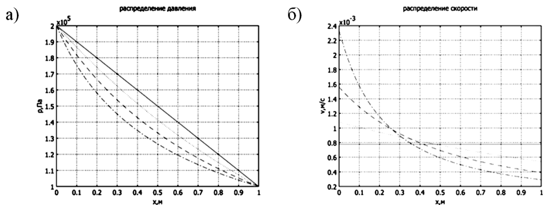
Рис. 6.26. Распределение давления и скорости на момент времени t = 1,0 с; сплошная линия -n = 0 ; пунктир -n = 1 ; штриховая линия -n = 2 ; штрих-пунктир -n = 3 .
