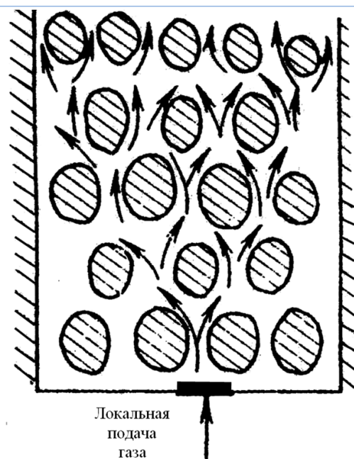
Рис.3.54. Рассеяние газа в мёрзлом грунтовом образце, подаваемого из локального источника (с использованием материалов [20]).
