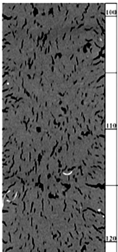
Рис. 2.4. Фрагмент рентгеноплотностного среза. Серое - осадок, чёрное – трещины, обусловленные дегазацией осадка (глубина 100-120 см) [Токарев и др., 2019].
