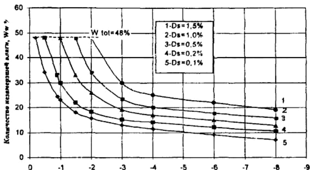
Рис. 5.19. Содержание незамерзшей влаги в мерзлой засоленной глине [Рекомендации..., 2001].
