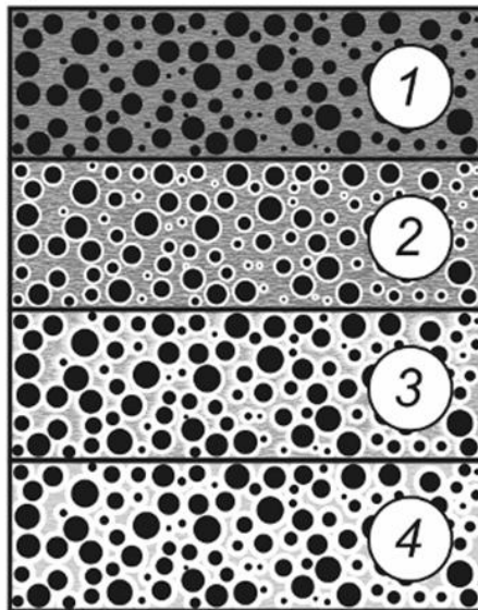
Рис. 3.1. Модель оттаивания мерзлой породы: схема расположения зон оттаивания, 1 – талая зона, 2 – оттаивающая зона, 3 – пластичномерзлая зона, 4 – твердомерзлая зона [Зарецкий, 1988].
