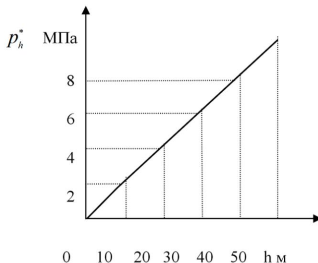
Рис. 5.12. Зависимость критического давления от глубины
