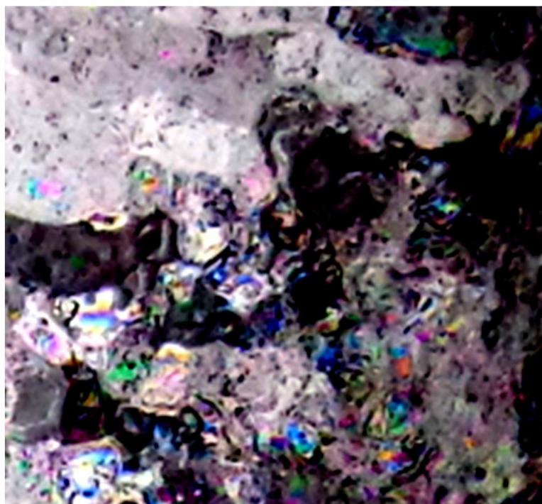
Рис. 3.26. Зона дробления и пластических деформаций. Съёмка в поляризованном свете. Фото А.Н. Хименкова.
