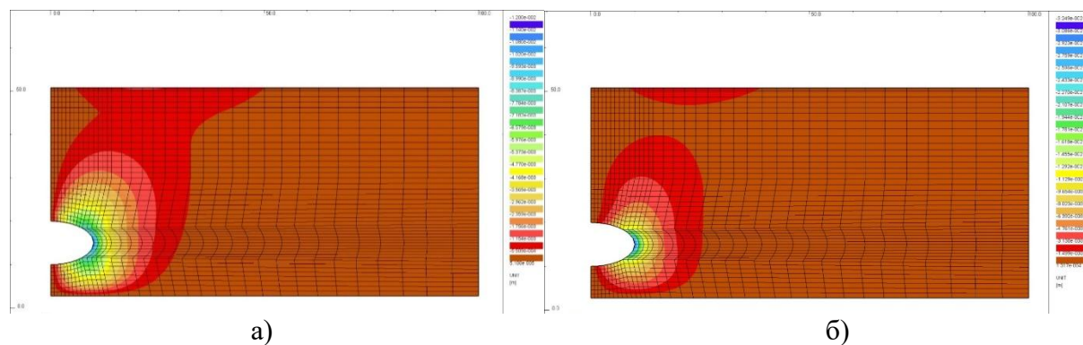
Рис.6.9. Этап 2. Зоны пластичности в модели Хоека-Брауна (а) и Друкера-Прагера (б).
