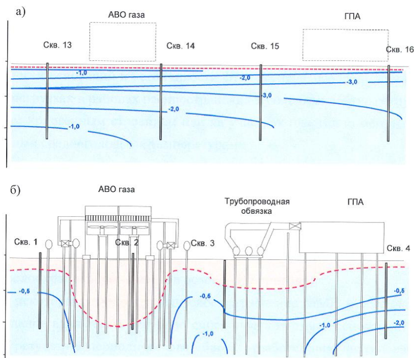
Рис. 5.20. Изменение температурного поля в основании сооружений Медвежьего газового месторождения: а) естественные условия (июнь 1978); б) техногенные талики после 5 лет эксплуатации август 1993) [Грива, 2006].
