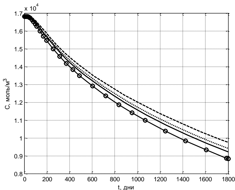
Рис. 6.37. Зависимость концентрации газа в фиксированной точке образца ( x_1=0.5 м, x_2=0.5 м) от времени для разных значений значений коэффициента D_s . Сплошная линия соответствует значению -D_s=D_k , штриховая -D_s=0.1D_k , пунктирная -D_s=10D_k . Рассматривалась нелинейная фильтрация по закону (5) и адсорбция по закону Генри с коэффициентом \kappa = 0.4 . Концентрация керогена равнялась 10%.
