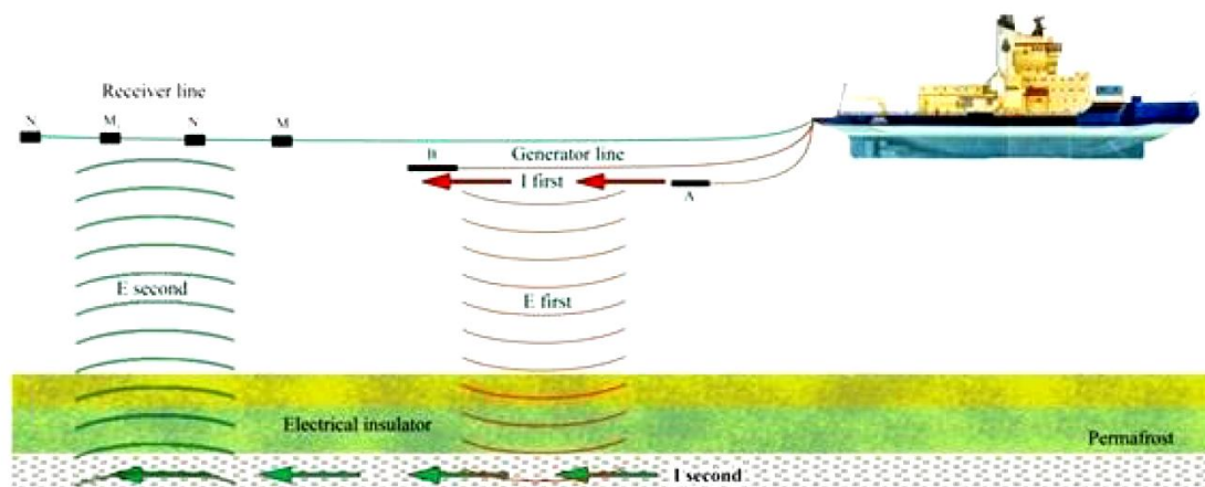
Рис. 7.7. Методика выполнения ЗСБ, ЧЗ на шельфе.
