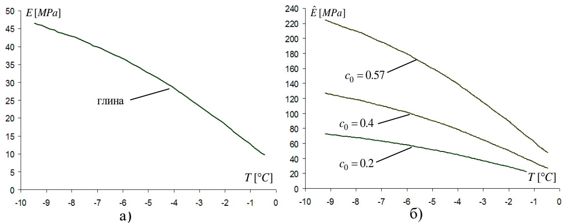
Рис. 6.7. Эффективные механические характеристики мёрзлых грунтов
