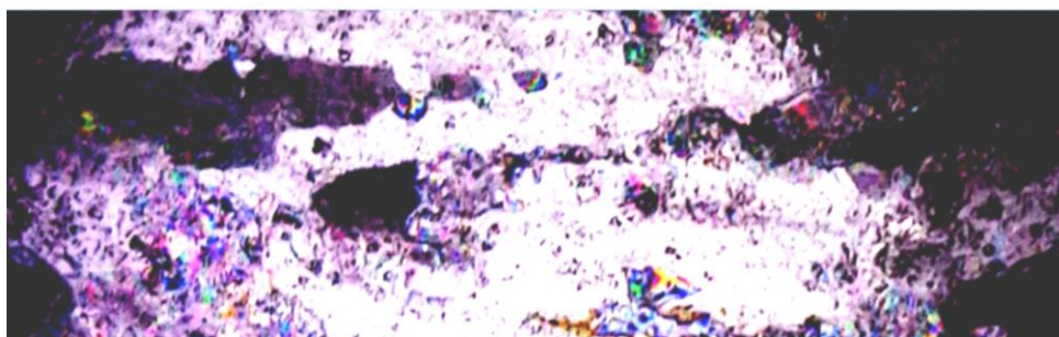
Рис. 3.27. Зона дробления и будинажа и пластических деформаций. Съёмка в поляризованном свете. Фото А.Н. Хименкова.
