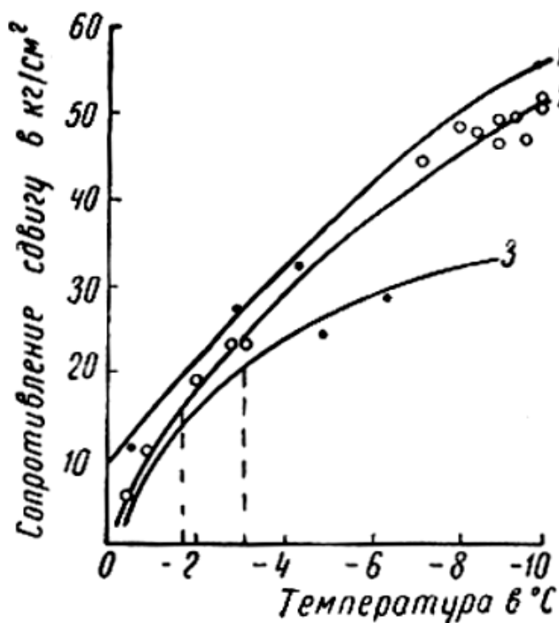
Рис. 3.3. Зависимость сопротивления сдвигу мёрзлого грунта и льда от температуры: а) 1 - лёд; 2 – супесь; 3 – глина [Велли и др., 1963].
