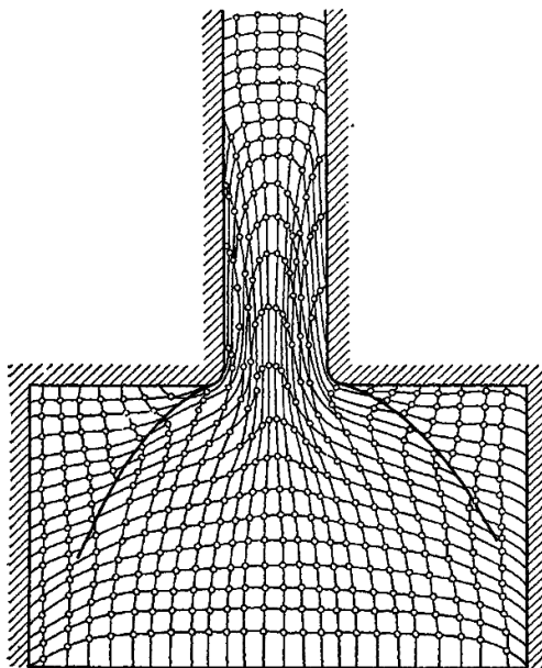
Рис. 4.69. Деформация прямоугольной сетки линий после проведения эксперимента по определению направлений главных деформаций в медленно движущейся пластичной массе, продавливаемой через узкое отверстие [Надаи, 1969].
