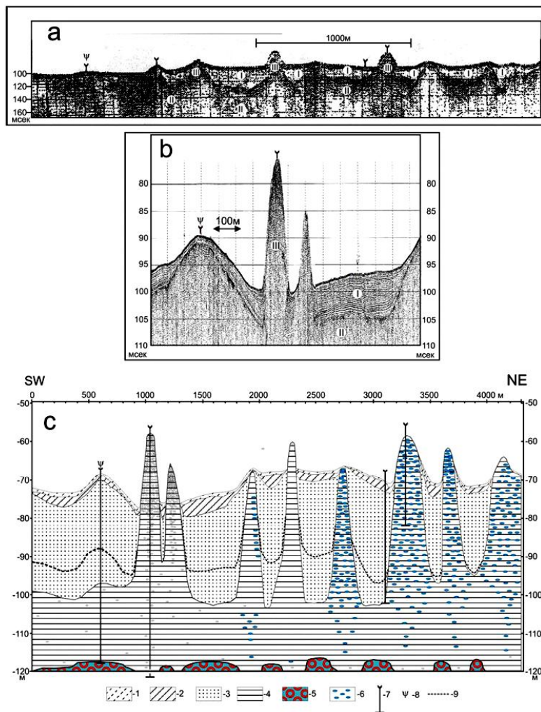
Рис. 2.10. Временные разрезы, полученные на объекте «Диапиры» и их интерпретация по данным бурения: а – временный разрез, полученный с помощью электроискрового источника (частоты 0,8-1.2 КГц), б – временной разрез импульсного профилографа (частота 3.5 КГц), с – интерпретация.
