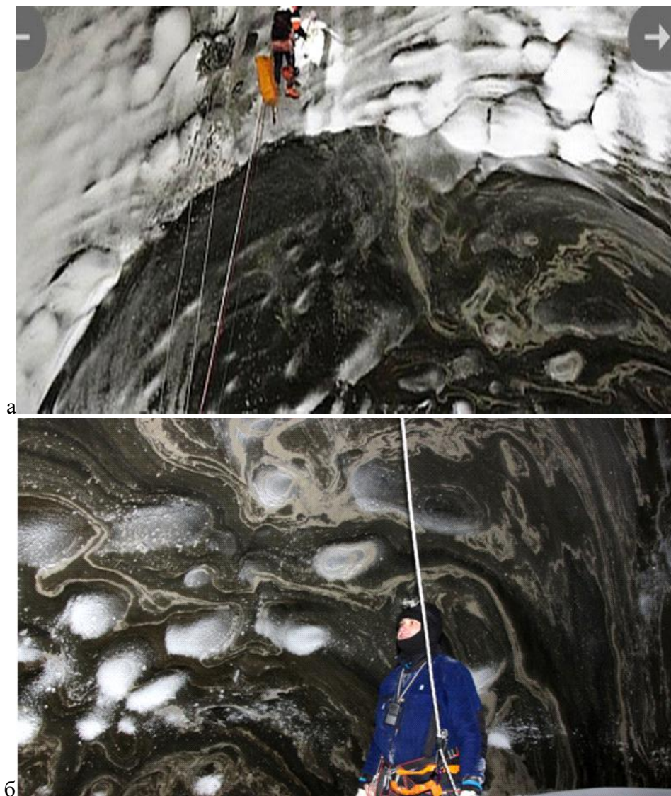
Рис. 4.45. Газовые флюиды в стенках грота в нижней части Ямальского кратера. а) зона контакта газовых флюидов с ячеистой структурой на стенке кратера; б) строение газовых флюидов (стенка грота). Фото В. Пушкарёва (ноябрь 2014г).
