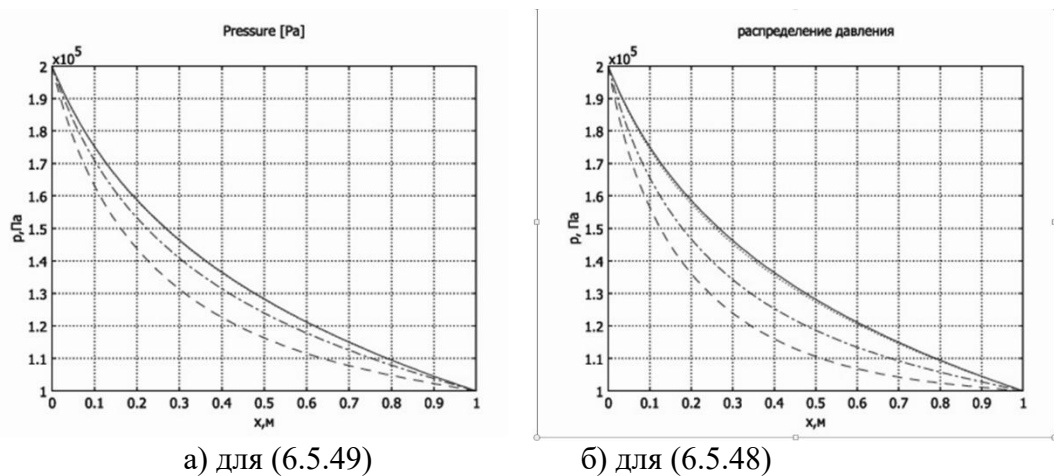
Рис. 6.22. Распределение давления: штриховая линия – t = 0,1 \text{с} ; штрих-пунктир – t = 0,2 \text{с} ; пунктир – t = 0,6 \text{с} ; сплошная линия – t = 1,0 \text{с} .
