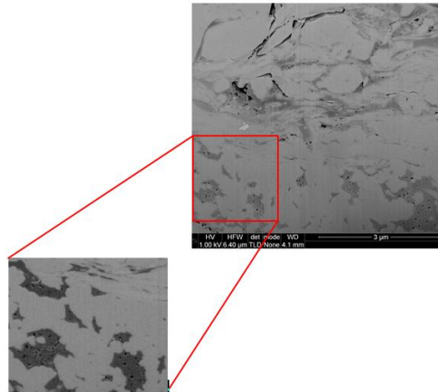
Рис.6.27. Двумерное изображение, полученное с помощью сканирующего электронного микроскопа [Ambrose R.J., Hartman R.C., Diaz-Campos M., Akkutlu I.Y., and Sondergeld C.H., 2012].
