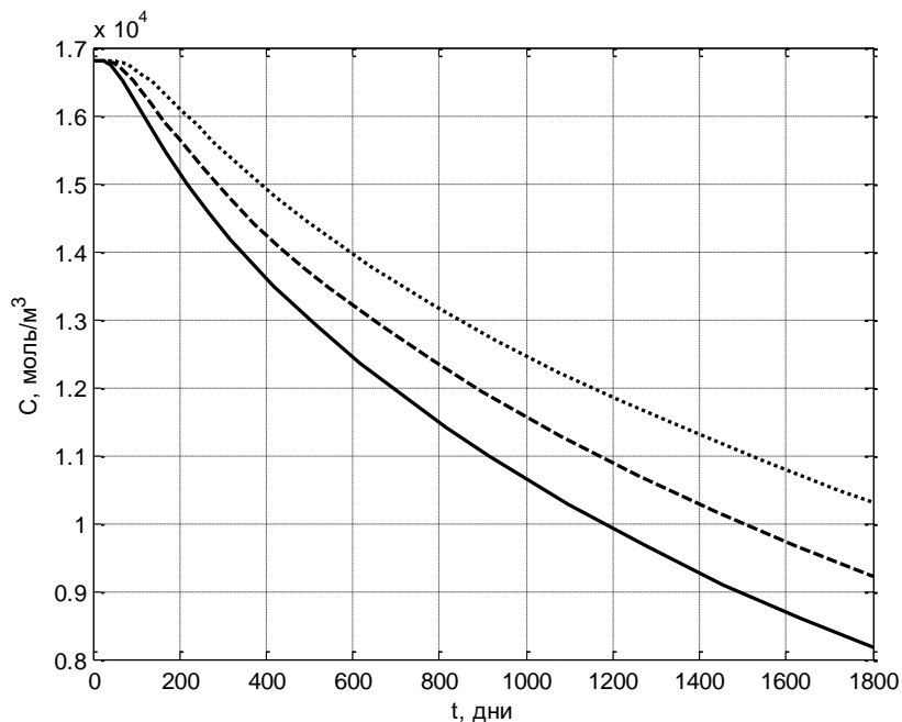
Рис. 6.33. Зависимость концентрации газа в фиксированной точке образца ( x_1=0.5\text{м} , x_2=0.5\text{м} ) от времени для разных значений концентрации керогена. Сплошная линия соответствует – 2% керогена, штриховая – 10%, пунктир – 25%. Рассматривалась нелинейная фильтрация по закону (5) и адсорбция по закону Генри с коэффициентом \kappa = 0.4 .
