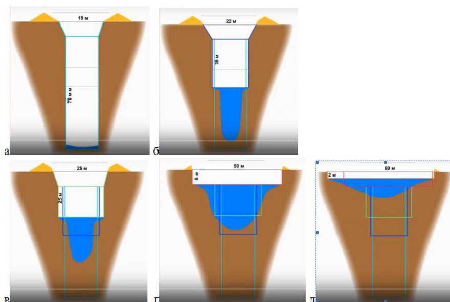
Рис. 4.4. Параметры озера сформировавшегося на месте Ямальского кратера: а – июль 2014, б – октябрь 2014, в – сентябрь 2015, г – октябрь 2016, д – сентябрь 2017.
