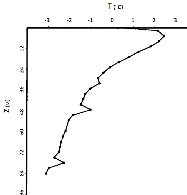
Рис. 3.9. Температурный профиль, в субаквальных осадках центральной, глубоководной части озера (глубина 4,5м) (скважина 78-10) [Burges et. al., 1982].
