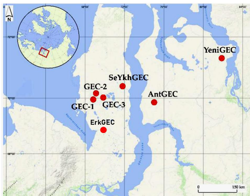
Рис. 4.2. Схема расположения ВГВ на севере Западной Сибири [Leybman et al., 2018] с добавлениями авторов.
