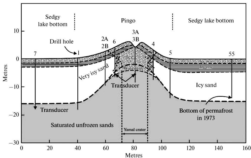
Рис. 5.16. Сопоставление размеров структурных элементов растущего гидролакколита (пинго) на Севере Аляски [Маскау, 1979] и Ямальского кратера [Leibman et al., 2014]
