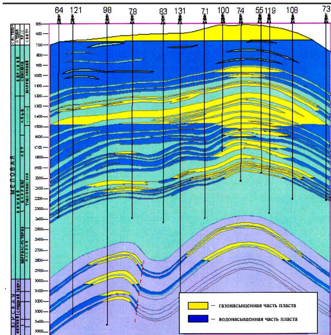
Рис. 1.26. Геологический разрез продуктивных толщ Бованенковского НГКМ (ВНИИГАЗ, 2003) Цитируется по [Грива, 2005].
