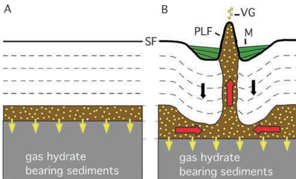
Рисунок 2.14. Схематический чертеж пингоподобной структуры (PLF) и рва окружающего её (M), связанных с разложением гидрата газа; VG – выход газа; SF – морское дно [Charles и др. 2007].
