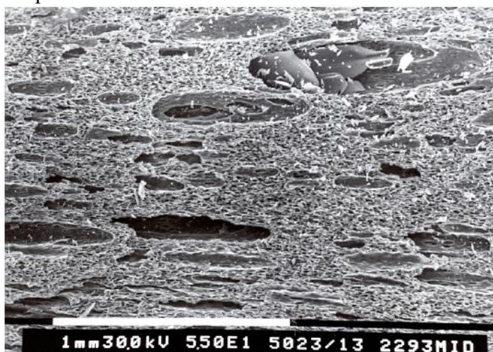
Рис. 5.13. Система вытянутых пор, микро и макротрещин в гранитном расплаве, формирующихся при быстром сбросе давления, скорость сброса 2500 атм/сек [Медведев и др., 2014].
