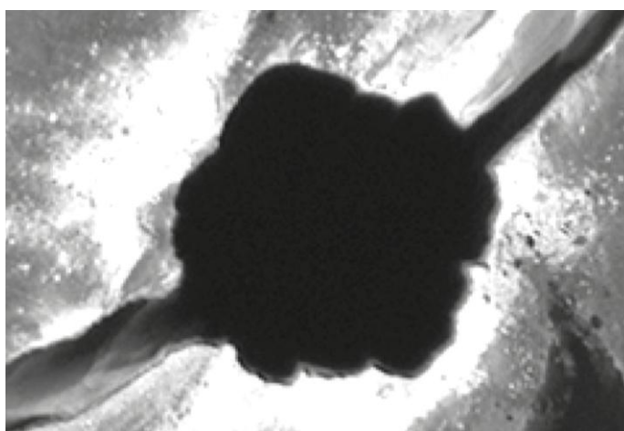
Рис. 4.21. Космоснимок водоёма, сформировавшегося на месте воронки газового выброса WV-1 20 июля 2018 г. [Богоявленский и др., 2019]
