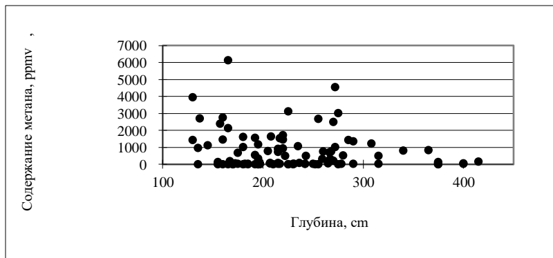
Рис. 1.14. Содержание метана в мерзлоте Якутии
