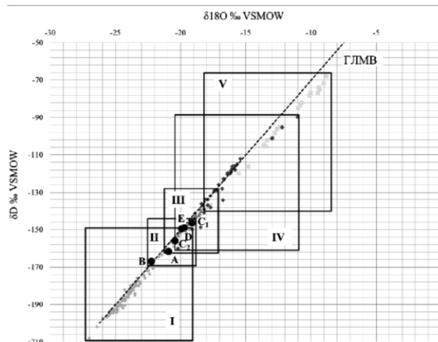
Рис. 9.14.. Изотопный состав подземных льдов в районе метеостанции Марре-Сале, подземных льдов воронки газового выброса и озерной воде в воронке. Диапазоны значений изотопного состава: I – полигонально-жильные льды неоплейстоценового возраста, Марре-Сале, II – пластовый лед из стенок воронки, III – слоистый пластовый лед, Марре-Сале, IV – полигонально-жильные льды голоценового возраста, Марре-Сале, V – пластовый стекловидный лед, Марре-Сале. Черными точками показаны значения изотопного состава льда стенок воронки и воды в озере. Буквы соответствуют горизонтам льда (А, В, С) и уровням воды в кратере: D – август 2014 г.; E – ноябрь 2014 г. ГЛМВ – глобальная линия метеорных вод [Стрелецкая и др., 2013].
