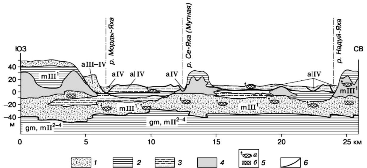
Рис. 1.25. Схематический разрез через Бованенковское месторождение [Стрелецкая, Лейбман, 2002]: 1 – пески; 2 – глины; 3 – переслаивание песков, суглинков и глин; 4 – пластовый лед; 5 – линзы криопэггов (а – установленные, б – предполагаемые); 6 – граница комплекса с пластовым льдом.
