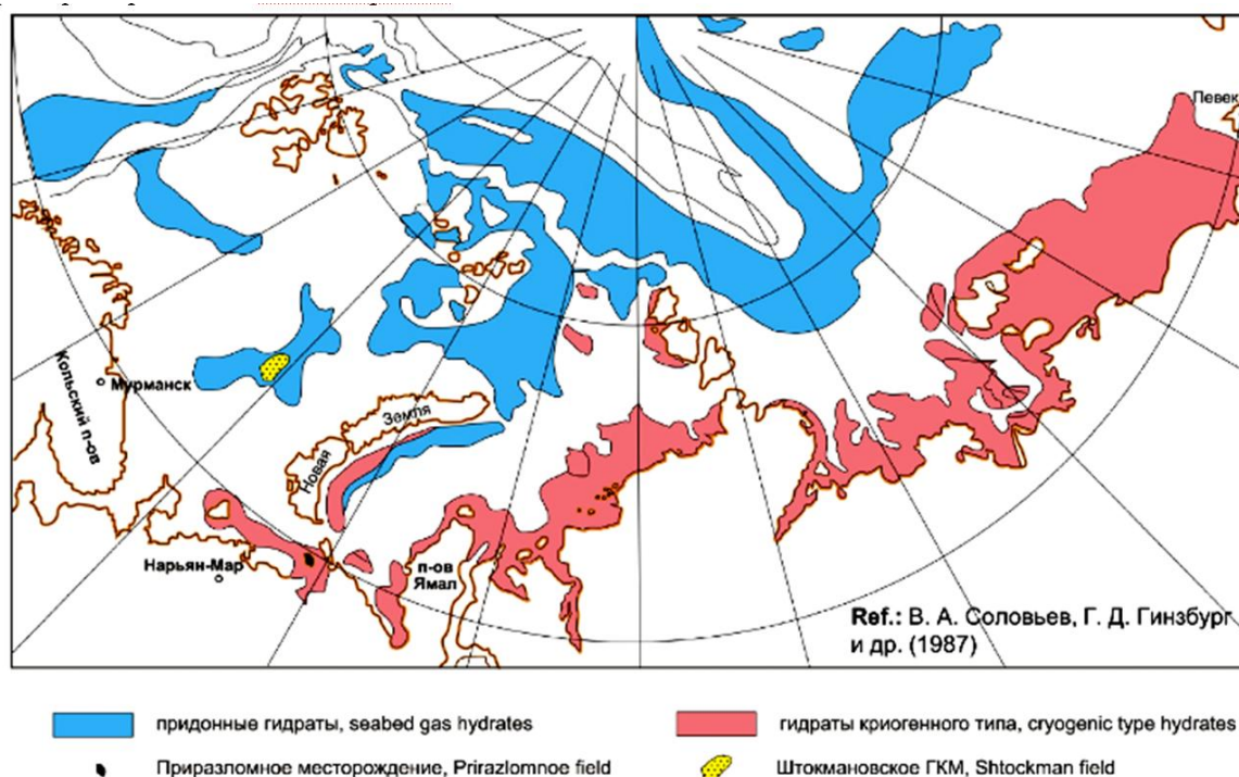
Рис. 2.11. Газогидраты и их распространение в Арктике [Соловьев и др., 1987].
