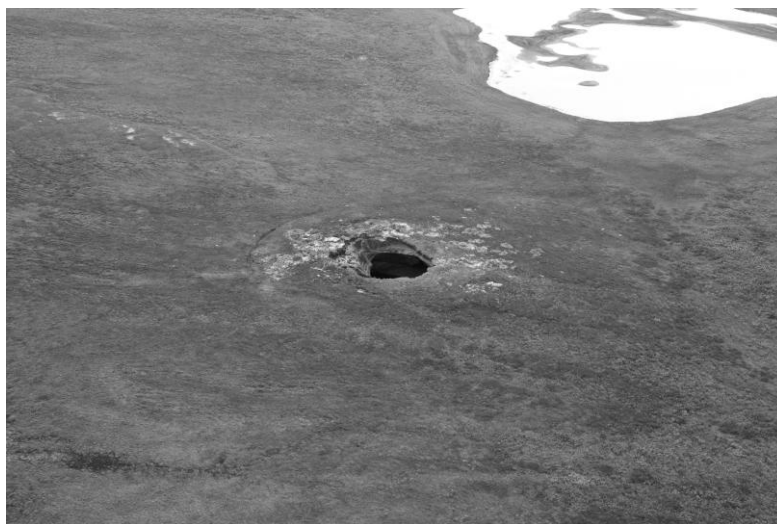
Рис. 4. 34. Воронка (п-в Ямал) дата съёмки 26. 07.13. (Фото А. Б. Осокина)
