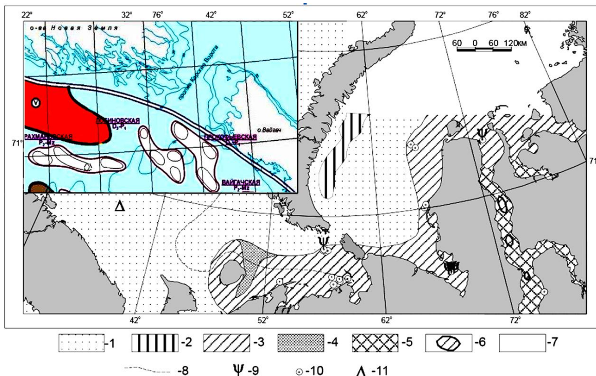
Рис. 2.9. Газонасыщенные осадки Баренцево-Карского шельфа [Рокос, 2008] (с добавлением фрагмента карто-схемы нефтегазоносных структур [Григоренко и др., 2011]).
