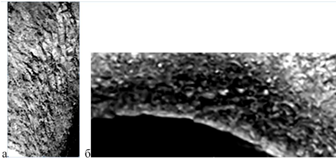
Рис. 4.67. Фрагменты криогенного строения глинистой толщи в стенке конусообразной части кратера. а) первичные сетчатые криотекстуры с преобладанием вертикальных шпиров; б) зона деформации (первичная слоистость осадков и шпирь льда смяты), примыкающая к стенке воронки.
