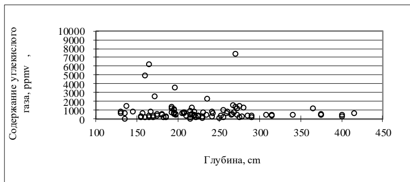
Рис. 1.15. Содержание углекислого газа в мерзлоте Якутии
