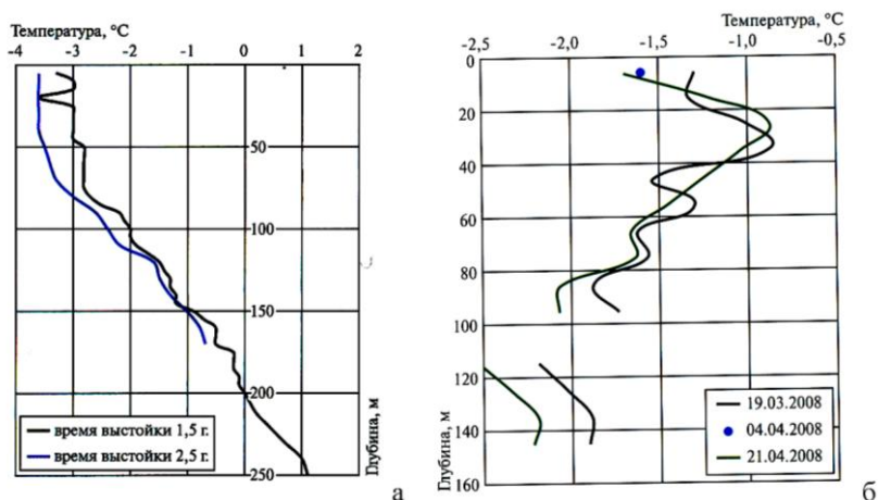
Рис. 3.10. Температура криогенной толщи под хасыреем на территории Бованенковского ГКМ а) III морская терраса; б) пойма [Криосфера..., 2013].
