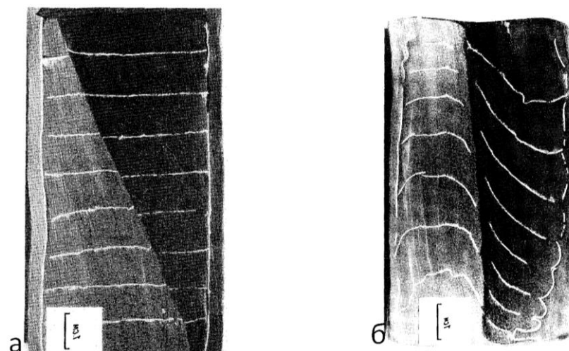
Рис. 4.71. Деформация при центрифугировании образца силикона разной плотности; более легкий (темный), более тяжелый (светлый). а - строение образца до центрифугирования; б - строение образца после центрифугирования [Лукьянов, 1989]
