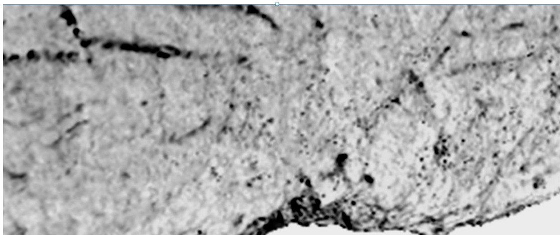
Рис. 3.41. Распределение газовых включений в нижней части образца. Фото А.Н. Хименкова
