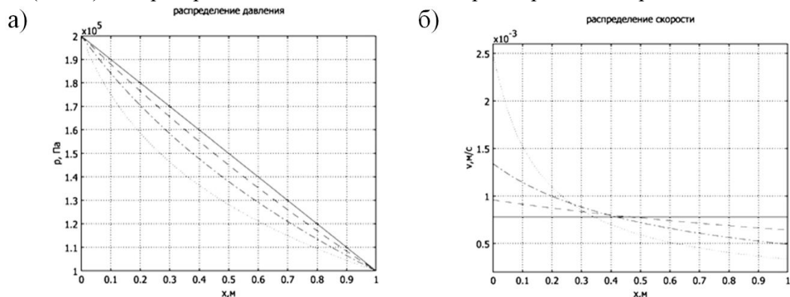
Рис. 6.25. Распределение давления и скорости на момент времени t = 1,0 \text{ с} ; сплошная линия -\beta = 0 ; штриховая линия -\beta = 0,4 \cdot 10^{-5} \text{ Па}^{-1} ; штрих-пунктир -\beta = 1,0 \cdot 10^{-5} \text{ Па}^{-1} ; пунктир -\beta = 2,0 \cdot 10^{-5} \text{ Па}^{-1} .
