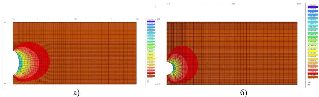
Рис.6.15 Этап 2. Горизонтальные смещения в модели Хоека-Брауна при 2a=b (а) и a=b (б).
