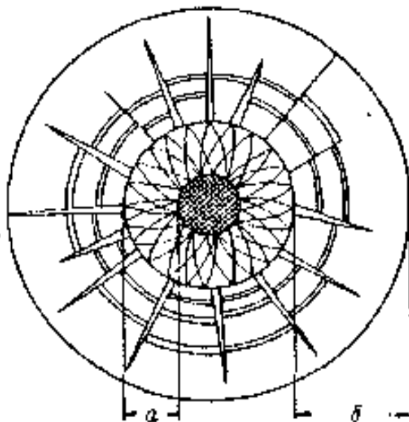
Рис. 5.5. Схема разрушения породы при взрыве [Покровский, 1980]).
