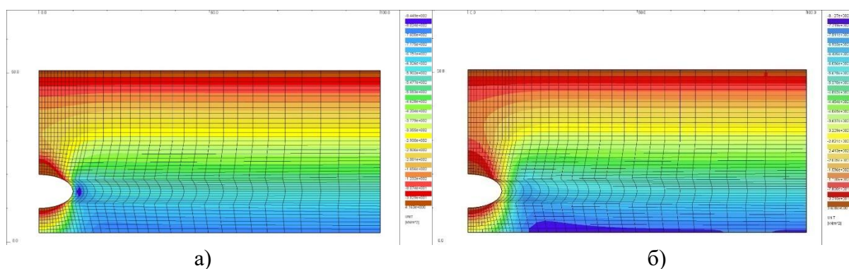
Рис.6.11. Этап 2. Вертикальная компонента напряжений в модели Хоека-Брауна (а) и Друкера-Праггера (б).
