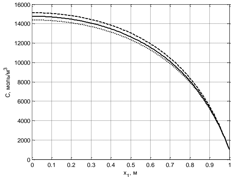
Рис. 6.38. Зависимость концентрации газа от координаты x_1 на фиксированный момент времени ( t=720 дней) для разных значений коэффициента D_s . Сплошная линия соответствует значению -D_s=D_k , штриховая -D_s=0.1D_k , пунктирная -D_s=10D_k . Рассматривалась нелинейная фильтрация по закону (5) и адсорбция по закону Генри с коэффициентом \kappa = 0.4 , концентрация газа в нанопорах равнялась 10%. Координата x_2 была фиксирована и равна x_2 = 0.5 м.
