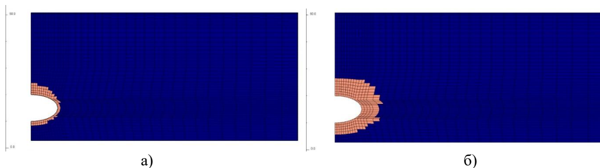
Рис.6.9. Этап 2. Зоны пластичности в модели Хоека-Брауна (а) и Друкера-Прагера (б).
