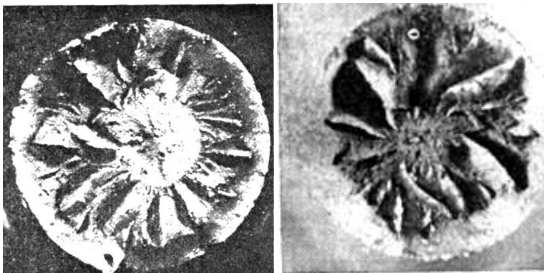
Рис. 5.9. Поверхность излома образцов стали после испытания на растяжение [Свидуневич и др., 2011].
