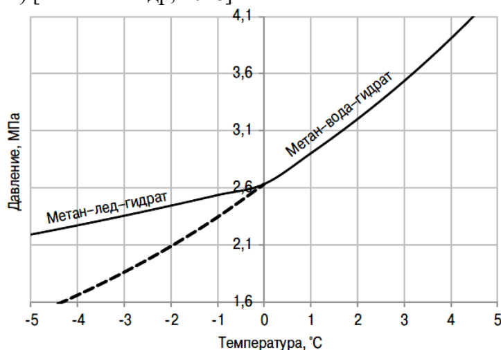
Рис. 3.12. Линии трехфазного равновесия «метан – вода – гидрат» и «метан – лед – гидрат». Пунктирная линия – метастабильное равновесие «метан – переохлажденная вода – гидрат» [Истомин и др, 2018].
