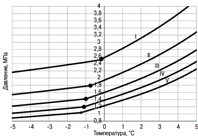
Рис. 3.13. Линии трехфазного равновесия «газ – вода (лед) – гидрат структуры I» для метана, диоксида углерода и их смесей. Состав газовой фазы: I – 100% \text{CH}_4 , II – 75% \text{CH}_4 + 25% \text{CO}_2 , III – 50% \text{CH}_4 + 50% \text{CO}_2 , IV – 25% \text{CH}_4 + 75% \text{CO}_2 , V – 100% \text{CO}_2 . Точки на линиях – четырехфазное равновесие «газ – вода – лед – гидрат» [Истомин и др, 2018].
