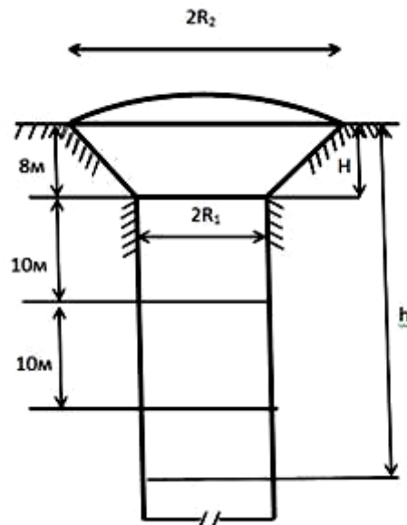
Рис. 5.11. Схема соотношения конической и цилиндрической частей Ямальского кратера
