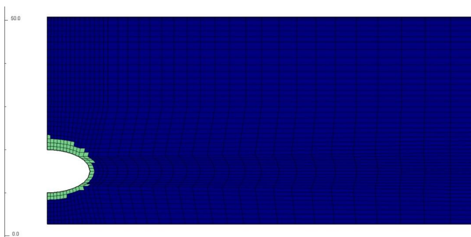
Рис.6.12 Этап 3. Зона пластичности в модели Хоека-Брауна.
