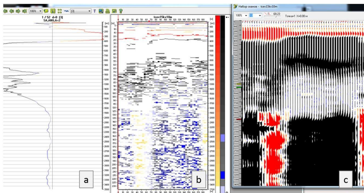
Рис. 7.8. Волновая форма (а), радарограмма в представлении «максмин» (б) и радарограмма сканов (с) профиля tcev15kv10m, пройденного к воронке, выполненного георадаром ГРОТ 12 в представлении программы GROT [Волкомирская, 2015].
