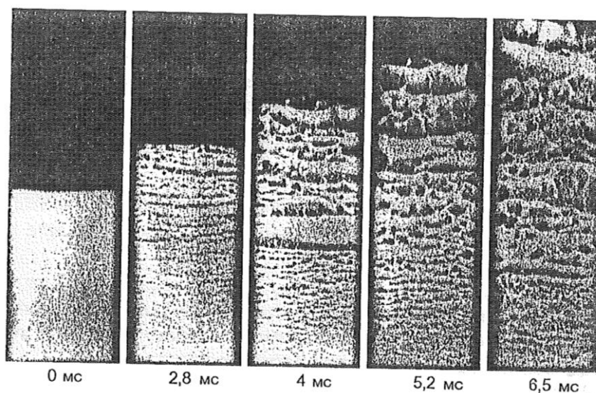
Рис. 5.14. Динамика слоя стеклянных шариков при быстром сбросе давления. [Кедринский, 2000].
