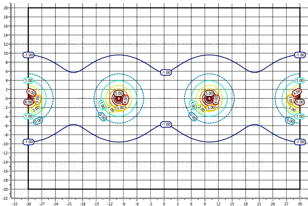
Рис. 5.18. Распределение теплового поля в грунте через 20 лет в 2D сечении в виде изолиний
