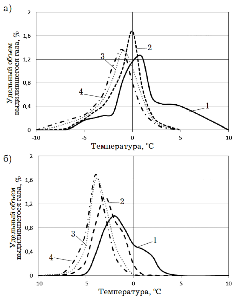
Рис. 3.53 . Зависимость объема газа, выделившегося под действием сжимающих нагрузок (1 - 0,001 МПа, 2 - 0,05 МПа, 3 - 0,1 МПа, 4 - 0,2 МПа) от температуры: а) пылеватый песок; б) суглинок [Карпенко и др., 2020].
