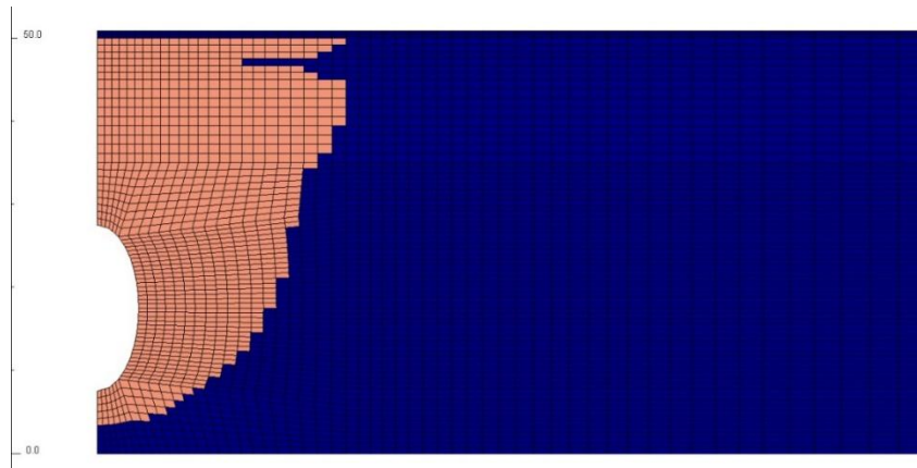
Рис.6.13 Этап 2. Зона пластичности.
