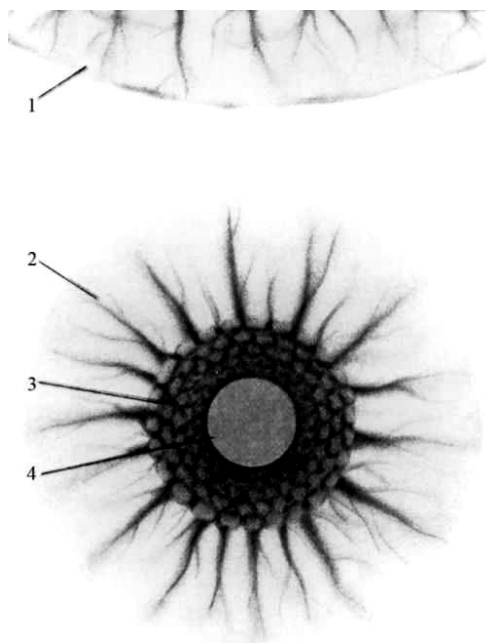
Рис. 5.5. Схема разрушения породы при взрыве [Покровский, 1980]).
