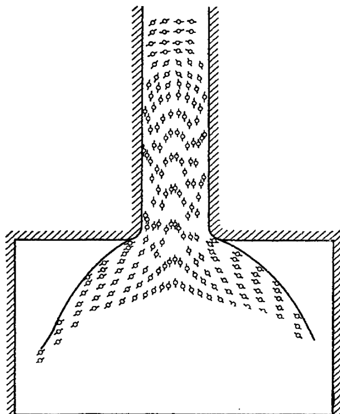
Рис. 4.70. Ориентация направлений главных деформаций в пластической массе, продавливаемой через канал [Надаи, 1969].
