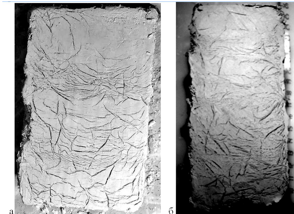
Рис. 3.38. Мерзлые образцы каолина. а – образец без газа; б – образец с газом. Фото. П. А. Соболева
