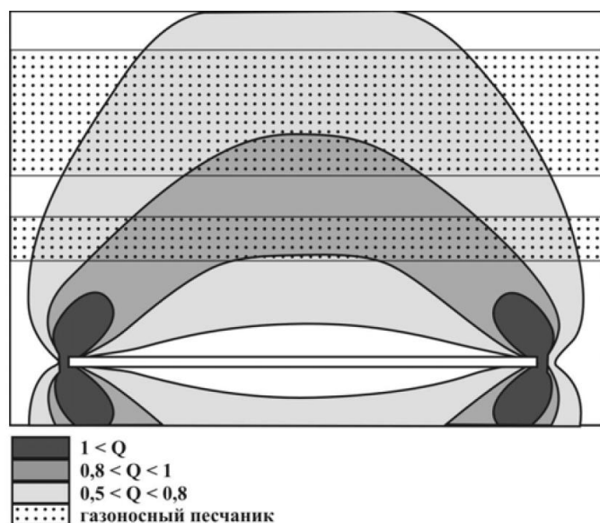
Рис. 4.72. Распределение параметра Q (объёмный дебит газа) [Круковская, 2004].
