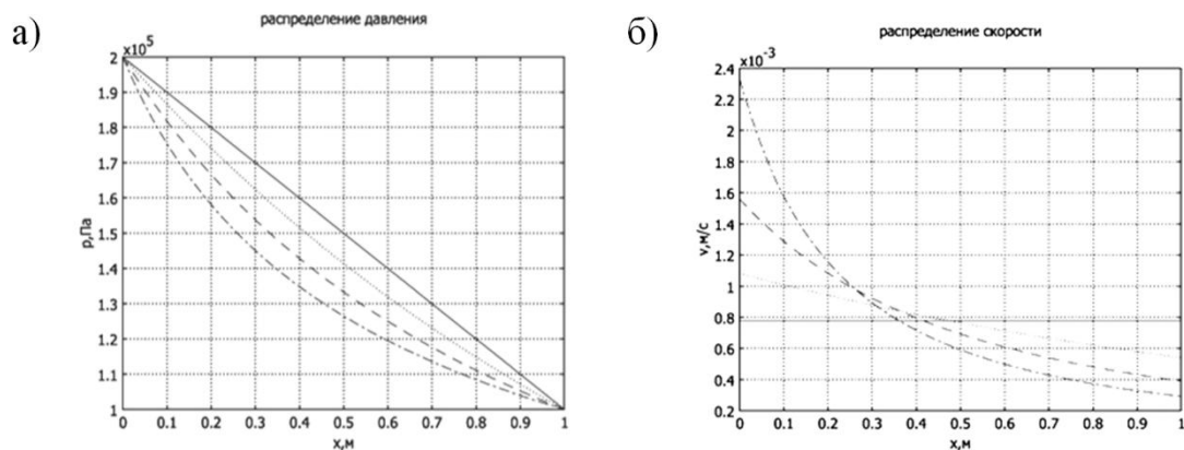
Рис. 6.24. Распределение давления и скорости на момент времени t = 1,0 \text{ с} ; сплошная линия -n = 0 ; пунктир -n = 1 ; штриховая линия -n = 2 ; штрих-пунктир -n = 3 .
