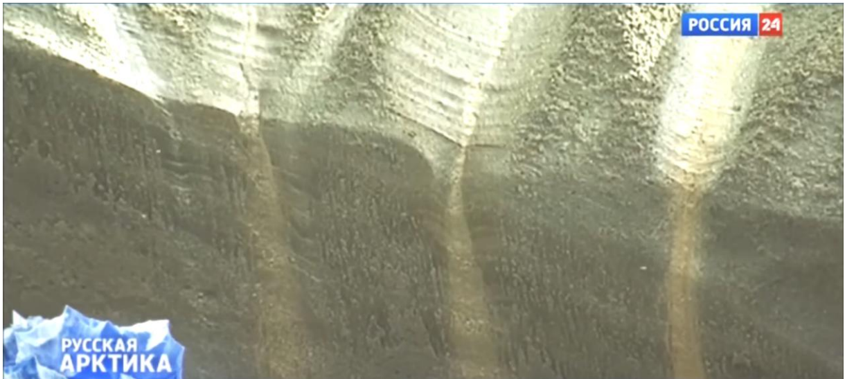
Рис. 4.46. Субвертикальная слоистость льда окаймляющего Ямальский кратер. Июль 2014. Скриншот видео.
