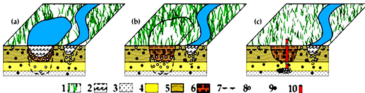
Рис.1.12. Палеоэкологическая реконструкция участка на Колымской пойме а) талые осадки под пойменным озером с потенциальным образованием метана; б) промерзание обогащенных метаном осадков после осушения озера; (с) метан, захваченный в порах и полостях мёрзлой породы после полного замерзания талика. 1 - пойма; 2 - речные и озерные воды; 3 – русловой гравийный слой; 4, речной аллювий, слой песка; 5, пойменный аллювий, иловый слой; 6 - озерные отложения, торфяные илы; 7 - граница вечной мерзлоты; 8, свободный метан; 9 - захваченный метан; 10, скважина 3,4-07 глубиной 25 м [Краев et al, 2017].
