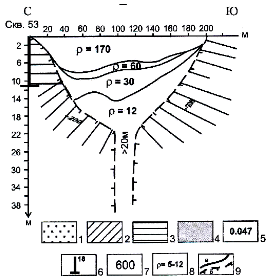
Рис. 5.25. Результаты донных геофизических работ на озере Средне-Ямальского ГКМ (данные В.М. Тимофеева и В.Б. Пугача 1982) 1-пески, 2-суглинки, 3-глины, 4-подземный лёд (ледогрунт), 5-озёрная вода, 6-скважина и её номер, 7-удельное сопротивление слоя, 8-криопэги, 9-границы а) слоёв с различным удельным сопротивлением, б)-мёрзлых пород. [Крицук, 2010].
