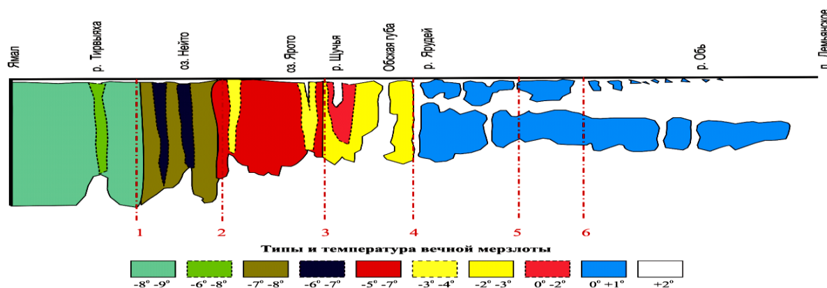
Рис. 3.7. Особенности влияния поверхностных водоёмов на температуру ММП Ямала [Бешенцев, 2009]
