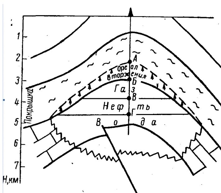
Рис. 3.55. Схема строения зоны аномально высокого пластового давления [Аникеев, 1971].
