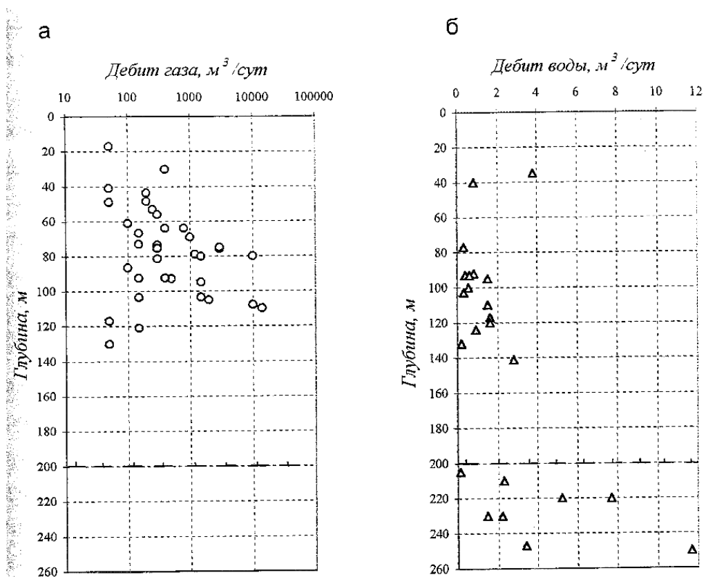
Рис. 1.24. Распределение газообразных (а) и жидких (б) флюидов по глубине мёрзлой толщи [Перлова, 2001].
