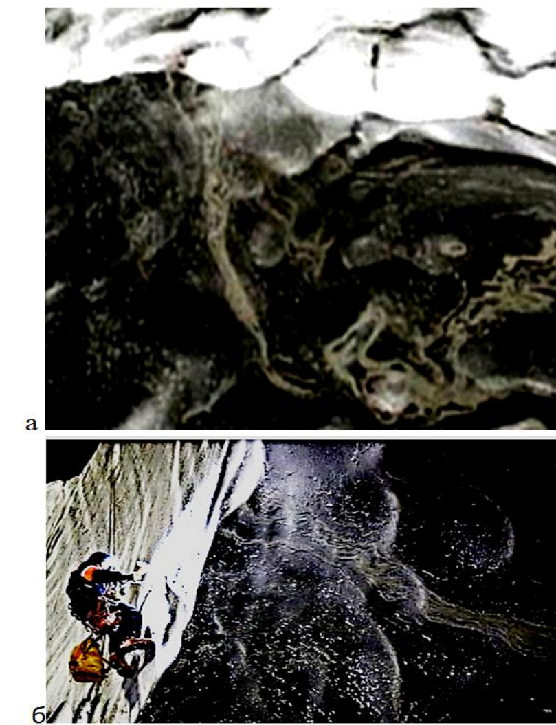
Рис. 6.5. Контакт газовых флюидов с ячеистыми льдами, соответствующими газовым пузырям на стенках Ямальского кратера. а – фрагмент рисунка; б – фото внутри грота. Ноябрь 2014. Фото В.А. Пушкарёва.
