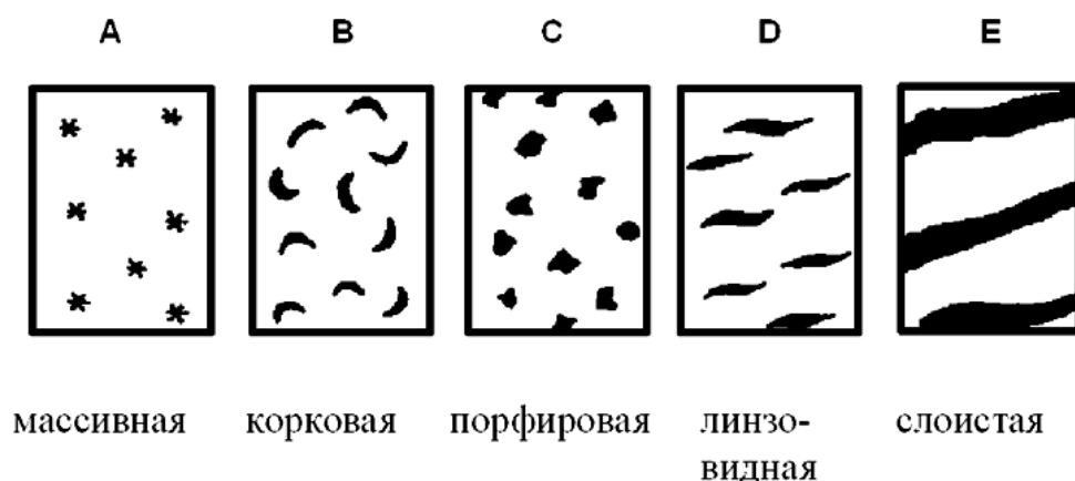
Рис. 1.10. Типы криогидратных текстур в мёрзлых породах [Якушев, 2009].
