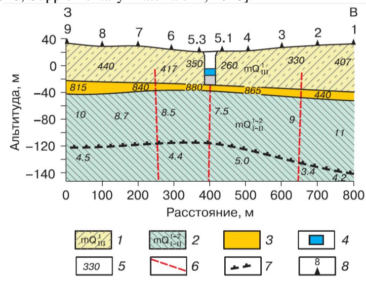
Рис. 4.40. Геологический разрез в районе Ямального кратера. 1– супеси и суглинки высокольдистые с пластовым льдом; 2 – суглинок, нижнесреднеплейстоценовые морские отложения ямальской серии; 3 – коллектор газогидратов; 4 – вода в кратере; 5 – удельное электрическое сопротивление пород; 6 – разлом; 7 – нижняя граница многолетнемерзлых пород; 8 – пункт измерения процесса становления электромагнитного поля [Оленченко и др., 2015].
