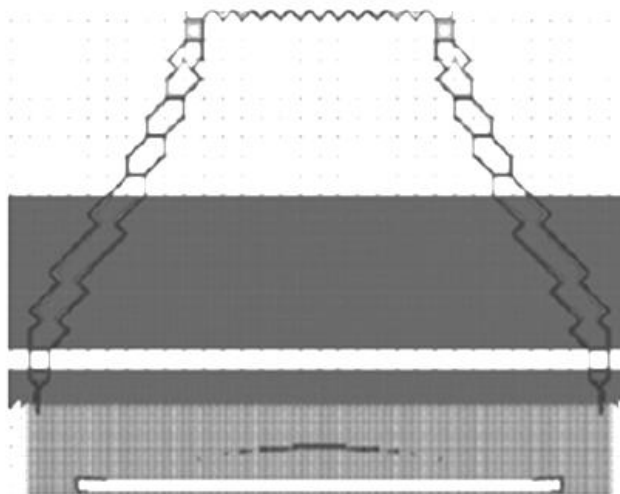
Рис. 4.73. Распределение расходов метана [Круковская, 2004].
