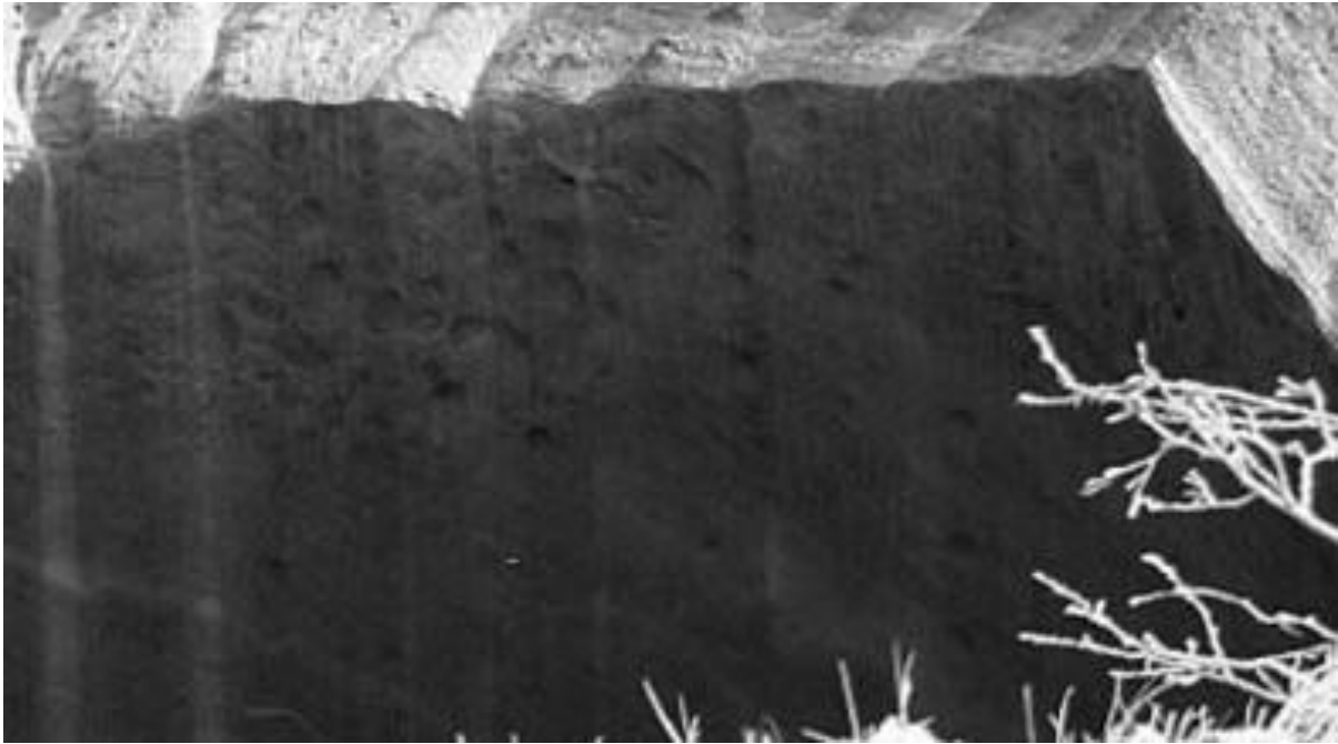
Рис. 5.10. Каверны на поверхности остатков свода. Фото В.А. Пушкарёва
