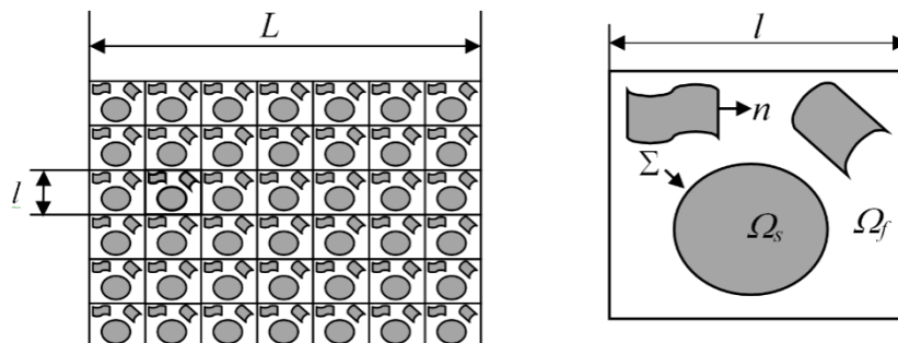
Рис. 6.19. Характерные масштабные уровни L и l : а) пористая среда с характерным размером L ; б) ячейка периодичности с характерным размером l .
