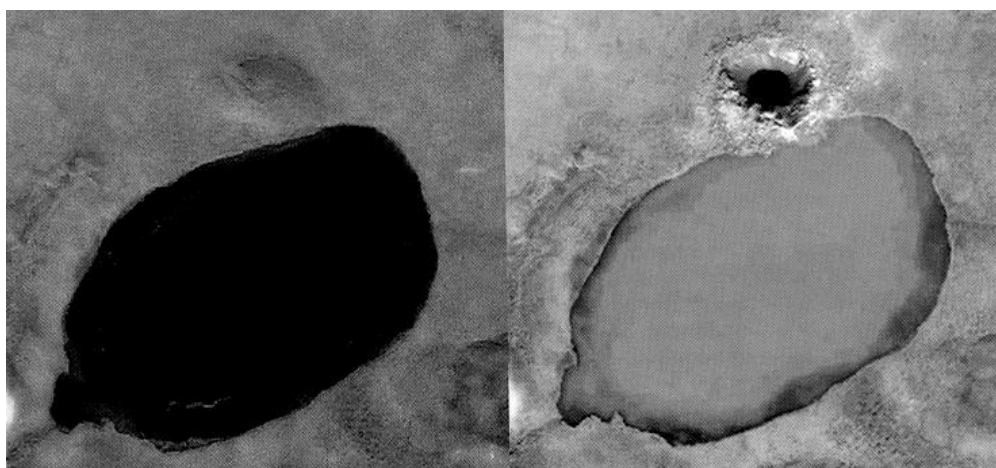
Рис. 4.23. Снимки территории формирования воронки газового выброса со спутника DigitalGlobe. а) 1 августа 2009 г., б) 19 июля 2013 г. [Богоявленский и др., 2016].
