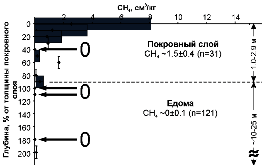
Рис. 1.13. Распределение средней концентрации метана по относительным глубинам в горизонте многолетнемёрзлых пород, оттаявшем в голоцене (покровном слое) в сводных разрезах почв Северо-Востока Сибири [Краев, Ривкина, 2017].
