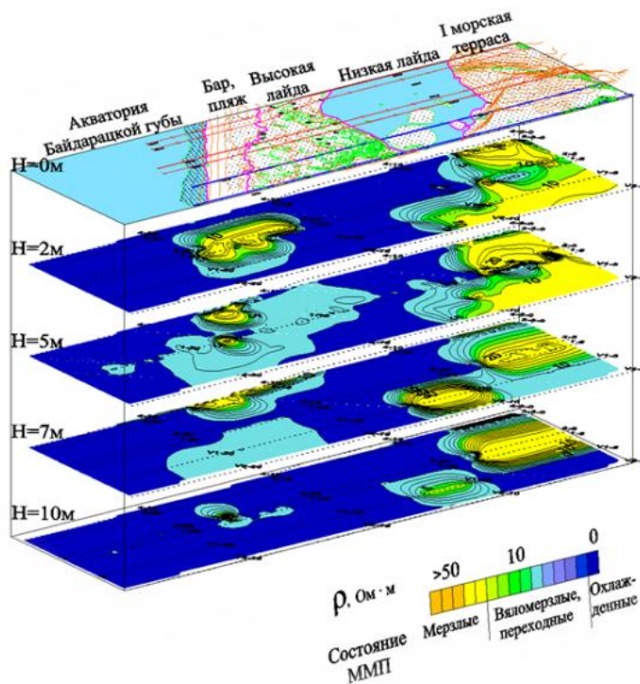
Рис. 2.1. Особенности строения криолитозны в районе Байдарацкой губы (Схема А.В. Кошурникова).
