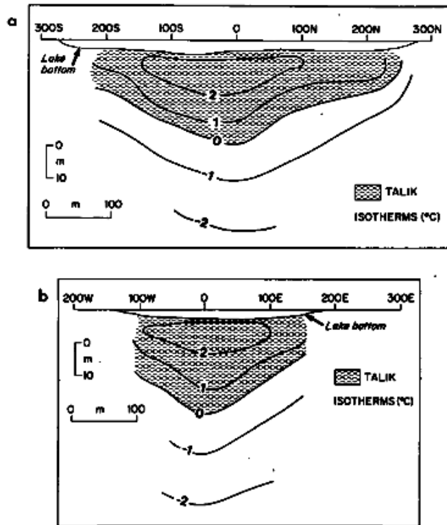
Рис. 3.8. Распределение температур субаквальных отложений оз. Иллисарвик (Канада) [Burges et. al., 1982].
