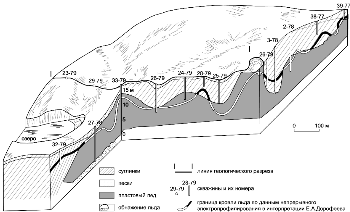
Рис. 1.23. Блок диаграмма останца третьей террасы на правобережье реки Сеяха [Пармузин, Суходольский, 1982].
