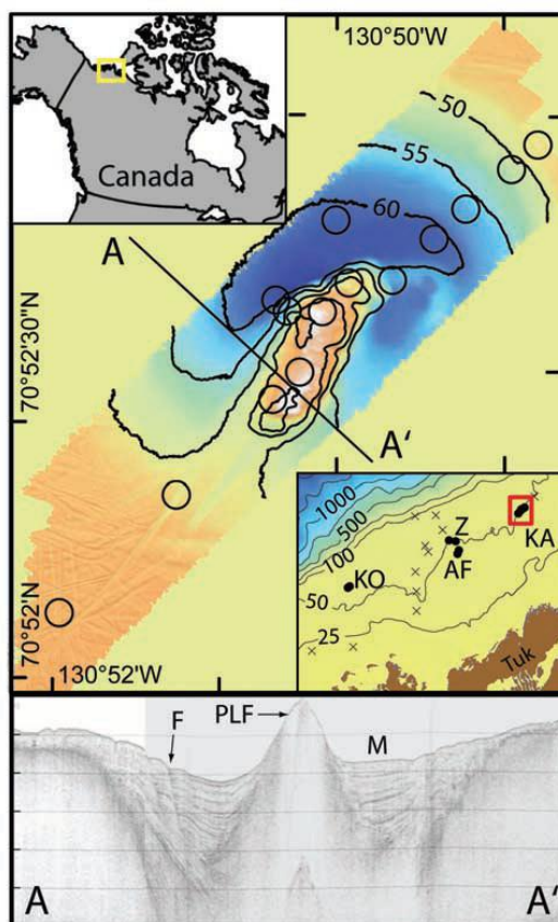
Рис. 2.13. Местоположения пингообразных бугров на морском дне (вверху). Положение сейсмического профиля (A-A 1 ) (внизу). PLF – пингообразный бугор, М – понижение, окружающее бугор заполненным слоистым слоем осадков, содержащих вертикально ориентированные трещины (F) [Charles и др. 2007].
