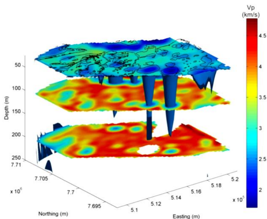
Рис. 3.11. Трёхмерное распределение областей пониженных скоростей под озерами по данным томографии [Majorowicz et al., 2015].
