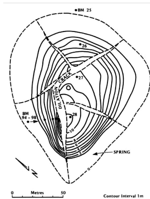
Рис. 5.2. Топографический план пинго №15 на полуострове Туктояктук (Аляска) [Маскау, 1979].
