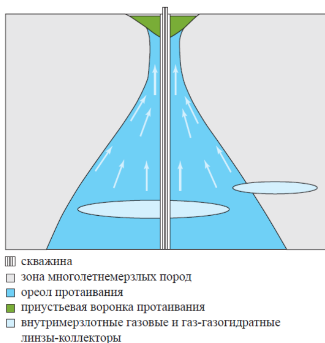
Рис. 5.17. Схема формирования потока внутримёрзлотного газа при оттаивании ММТ вокруг работающей скважины [Аветов и др. 2018].
