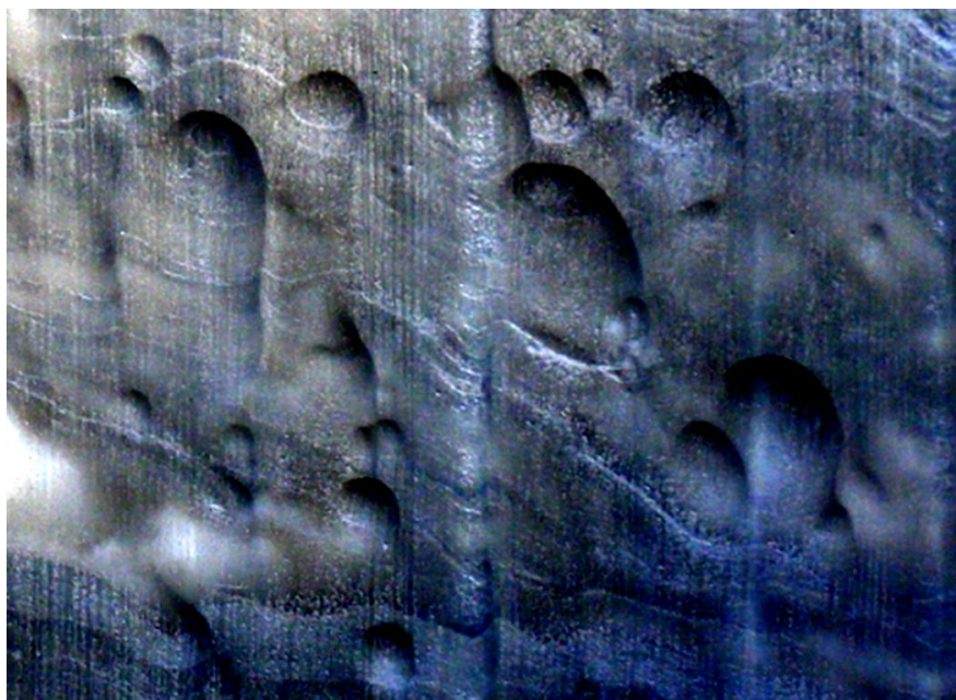
Рис. 4.51. Морфология газовых ячеек в стенках Ямальского кратера.
