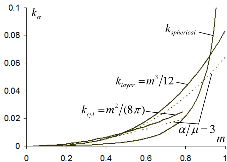
Рис. 6.18.. Проницаемость в пористой и трещиноватой среде.
