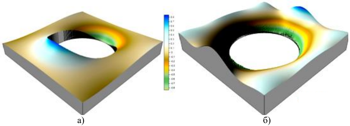
Рис. 6.20. Распределение псевдодавлений (а) и псевдоскоростей (б) в ячейке с включением радиуса R = 0.3 .
