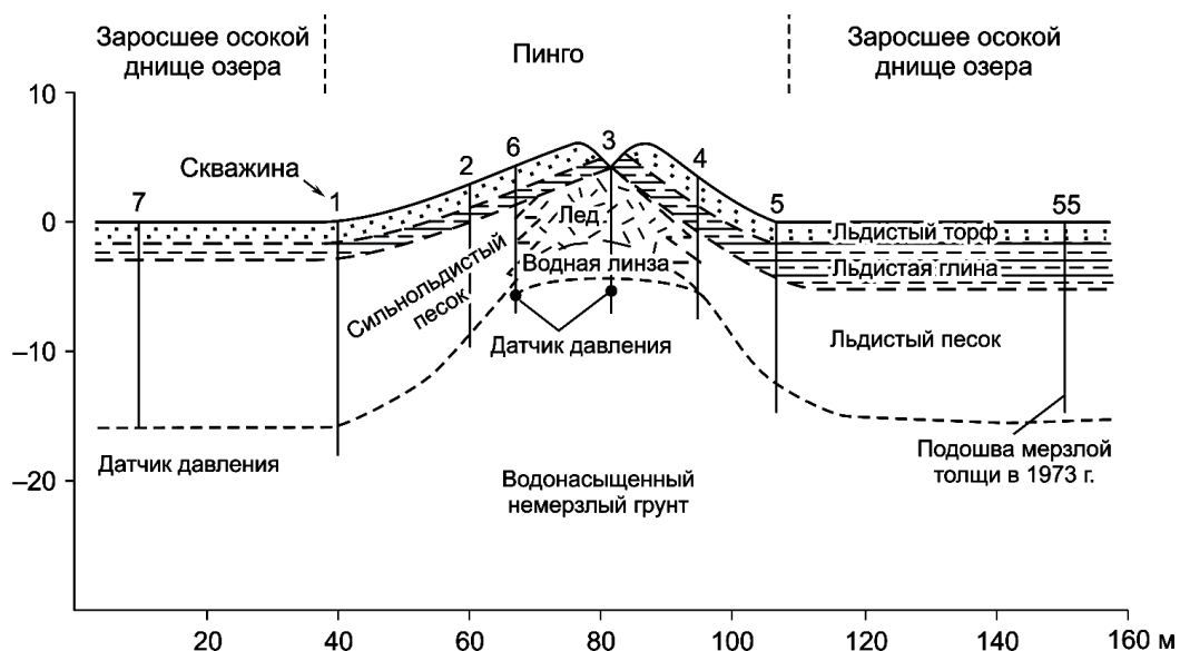
Рис. 1.16. Схема строения растущего пинго на Севере Аляски [Маскау, 1979].
