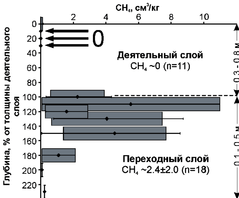
Рис. 1.11. Распределение средней концентрации метана по относительным глубинам в деятельном слое и периодически оттаивающем верхнем горизонте многолетней мерзлоты (переходном слое) в сводных разрезах почв Северо-Востока Сибири [Краев, Ривкина, 2017].
