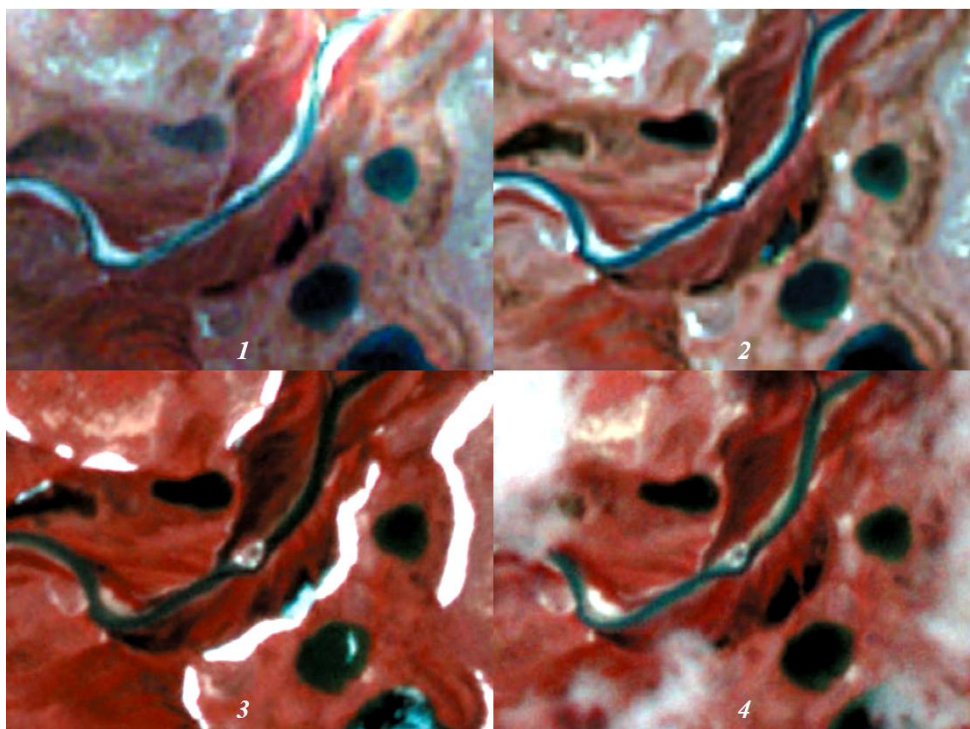
Рис. 4. 20. Космоснимки площади выброса газа: Sentinel-2 4 сентября 2015 г. и 17 июня 2016 г., (1 и 2), PlanetScope, 18 и 27 июня 2017 г., (3 и 4) [Богоявленский и др., 2019]
