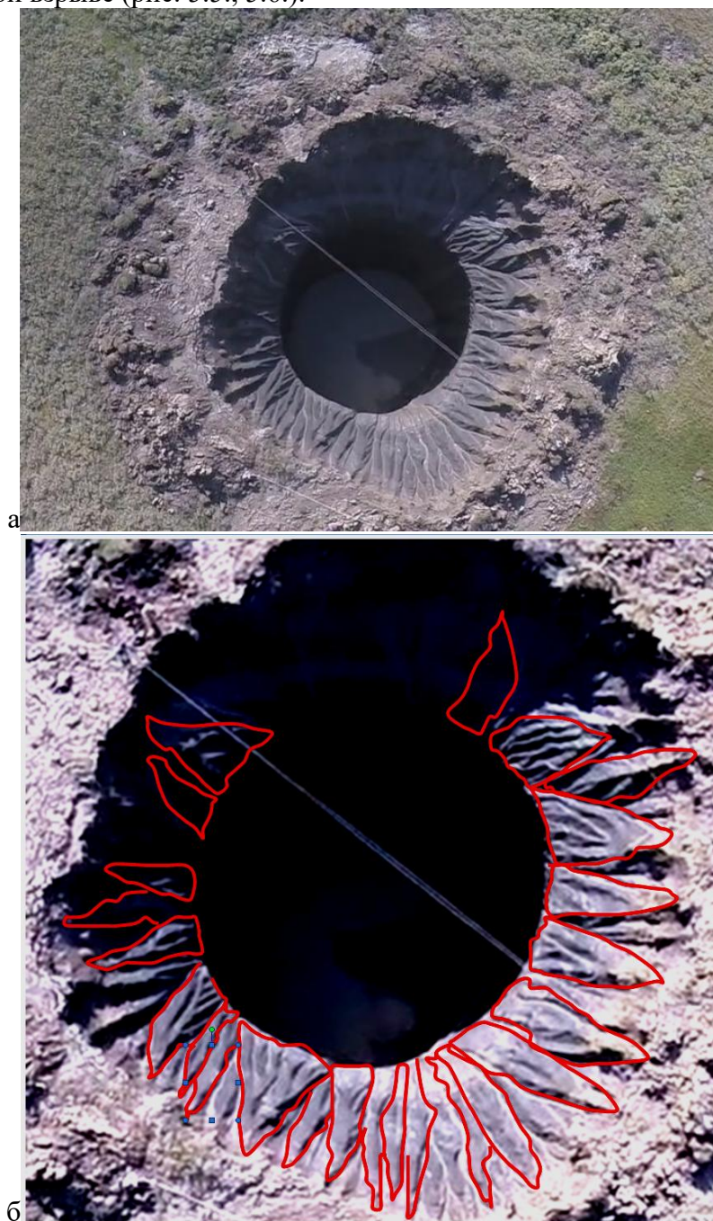
Рис. 5.7. Ямальская воронка вид сверху: а – фотография воронки; б – фотография с нанесёнными контурами неровностей поверхности конусообразной части воронки, соответствующими деформациям, возникшим при взрыве. Фото В. А. Пушкарёва
