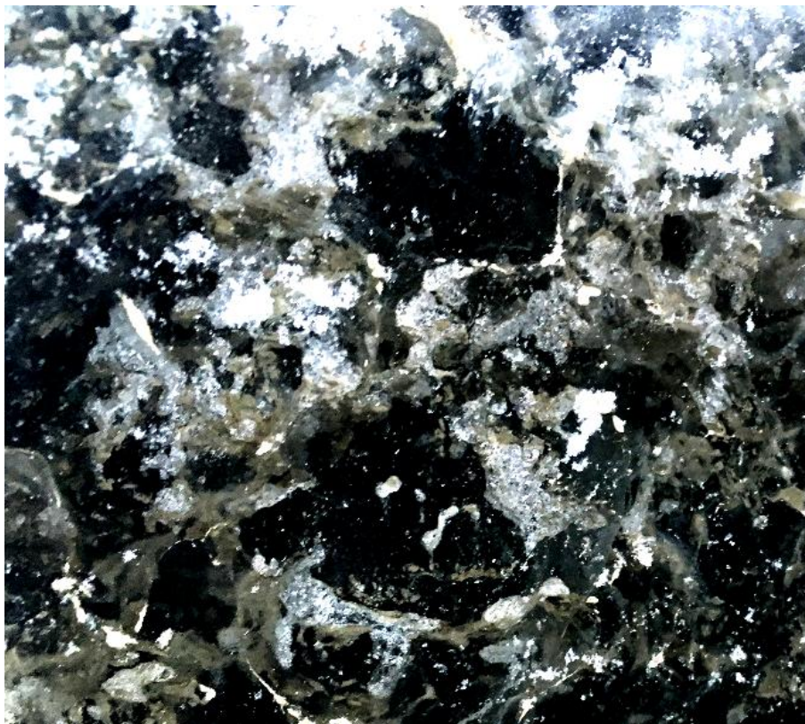
Рис. 1.3. Газовые скопления в виде гроздьев, лёд в стенке воронки газового выброса на реке Еркутаяха (Южный Ямал) Фото Ю. Станиловской.
