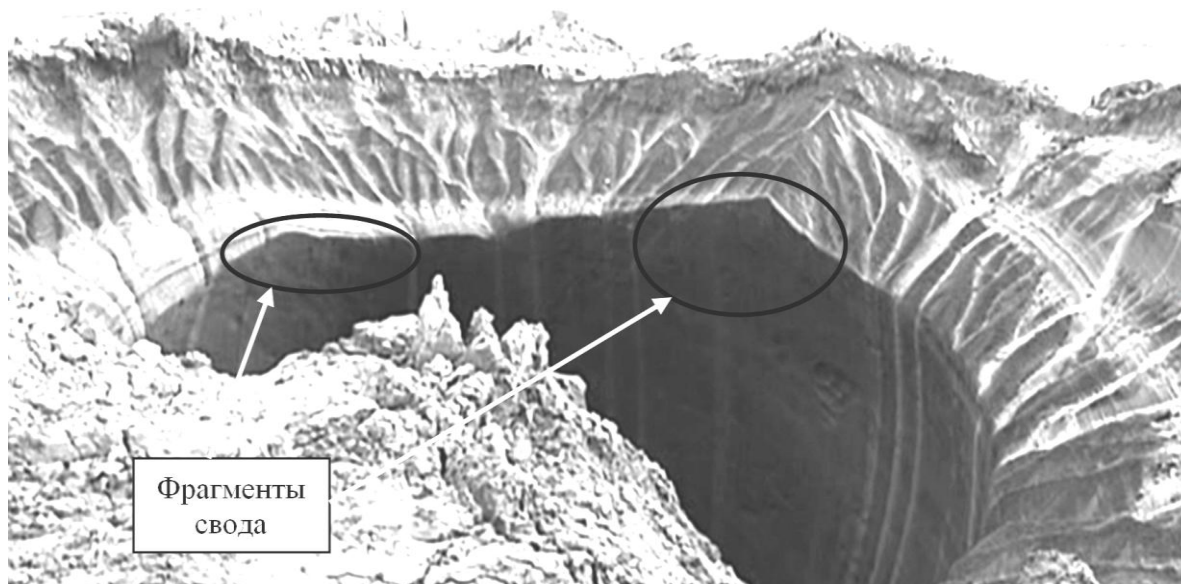
Рис. 4.62. Ямальский кратер. Фрагменты свода над газонасыщенной зоной, оставшиеся после выброса. Фото В.А. Пушкарёва, июль 2014.
