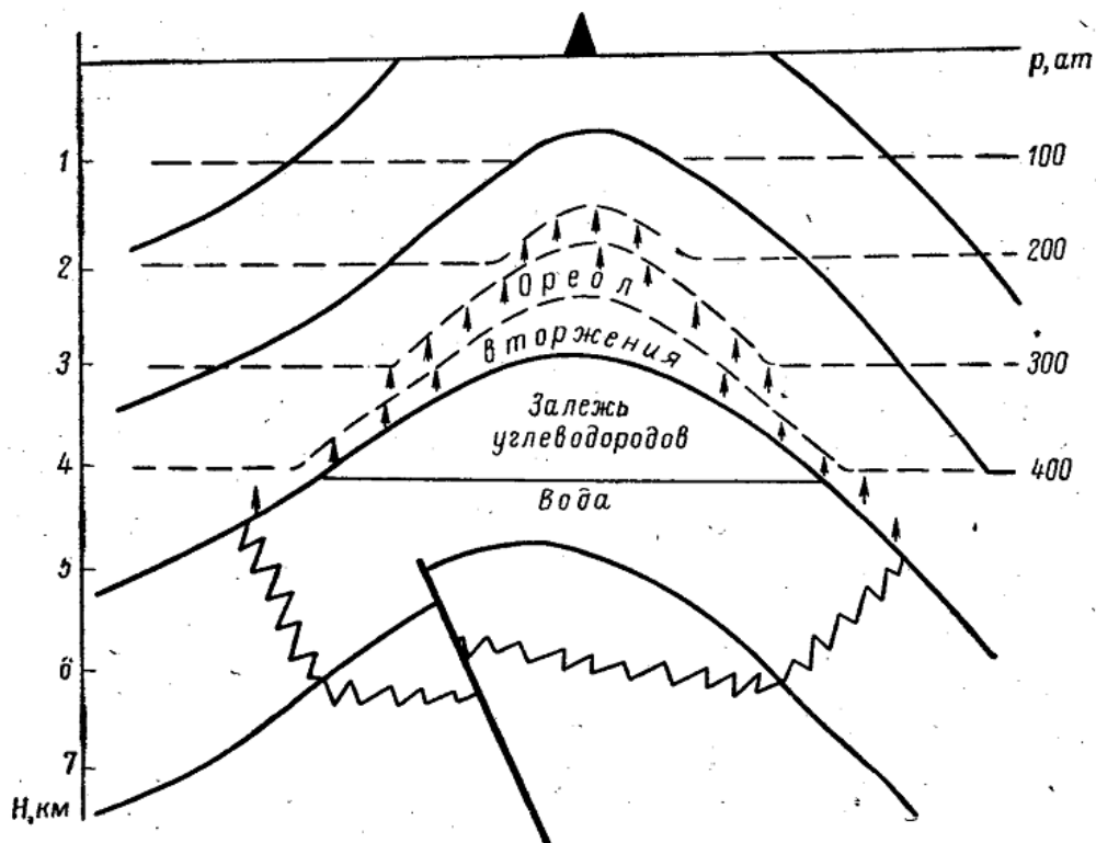
Рис. Распределение повышенных поровых давлений в ореоле вторжения над углеводородной залежью [Аникеев, 1979].
