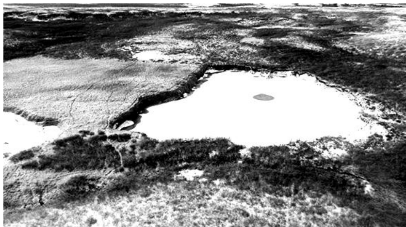
Рис. 4. 5. Озеро на месте Ямальской воронки Фото М. О. Лейбман Архив Института криосферы https://ria.ru/science/20171207/1510311618.html
