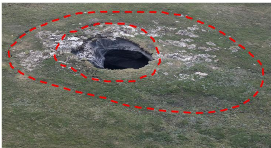
Рис. 3. 35. Концентрические трещины сформированные вокруг воронки (Фото А. Осокина).
