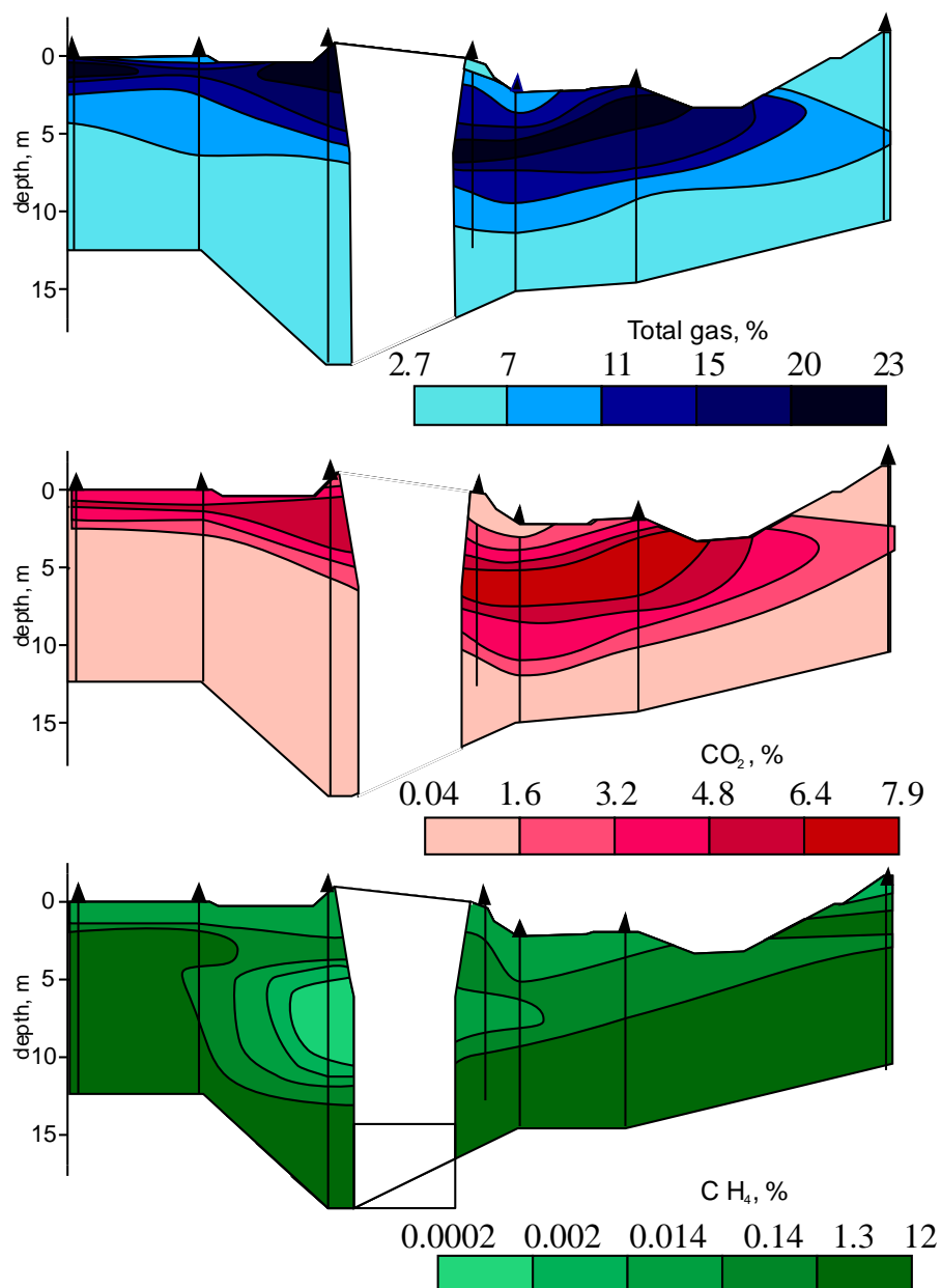
Рис. 4.36. Содержание газа в подземном льду [Supplementary Materials..., 2018]. Общая концентрация газа представлена в % при нормальных условиях, нормированных к объему подземного льда. Для CO 2 и CH 4 – в % в газовой смеси при нормальных условиях. Судя по результатам анализа содержания газа мощность подозёрного талика, не превышала 10-15 м. Ниже породы оставались в мёрзлом состоянии. Промерзание талика и дало наблюдаемую картину. Линза льдистой слоистой мёрзлой породы, с повышенным содержанием углекислого газа, соответствующая талику под озером вложена в массив с повышенным содержанием метана.
