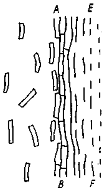
Рис. 5.24. Рассредоточенное разрушение на фронте выброса [Петухов, Линьков, 1983].
