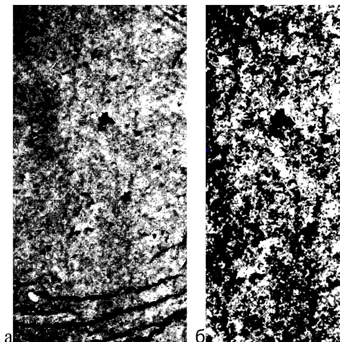
Рис. 3.35. Фотография слоя массивной криотекстуры (слой 3) после обработки: а – фото всего слоя, в нижней части фотографии горизонтальные шлиры льда (слой 2); б – увеличенный фрагмент. Фотография в отражённом свете. Фото. А.Н. Хименкова.
